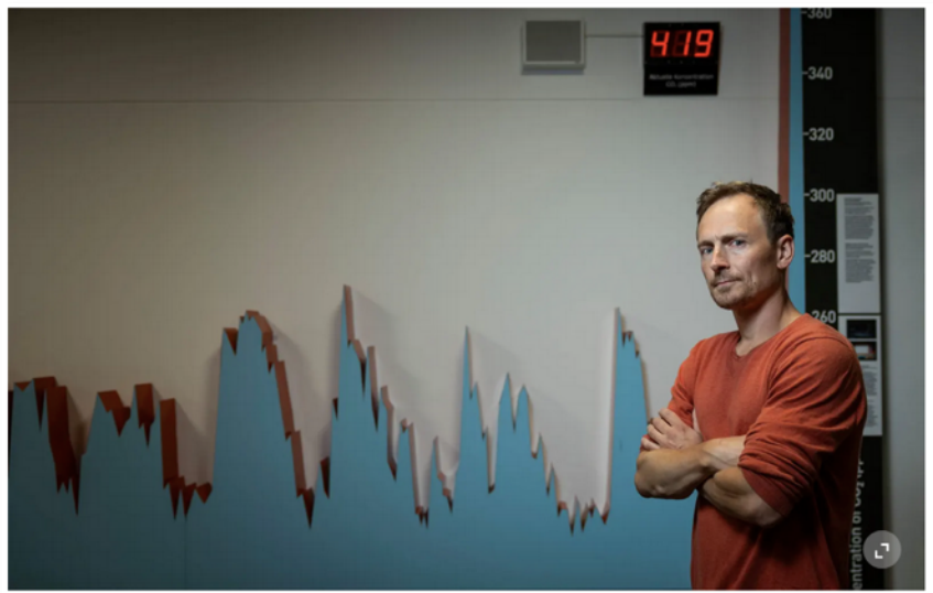
Klimaforscher Johannes Sutter im Oeschger-Zentrum der Uni Bern. Im Hintergrund sieht man die explodierende CO 2 -Kurve (aktuell bei 419 ppm CO 2 ). Foto: Beat Mathys
